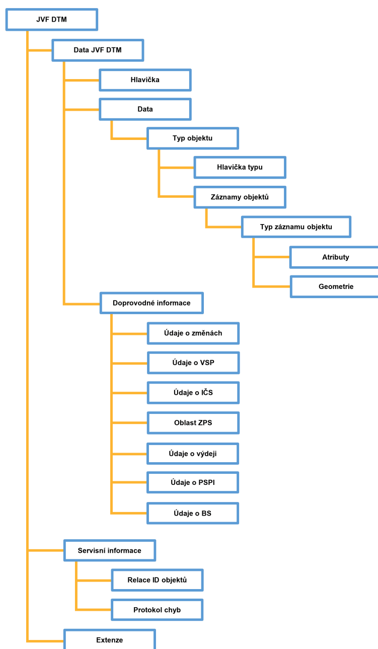
Obrázek č. 1: Struktura XML dokumentu JVF DTM
