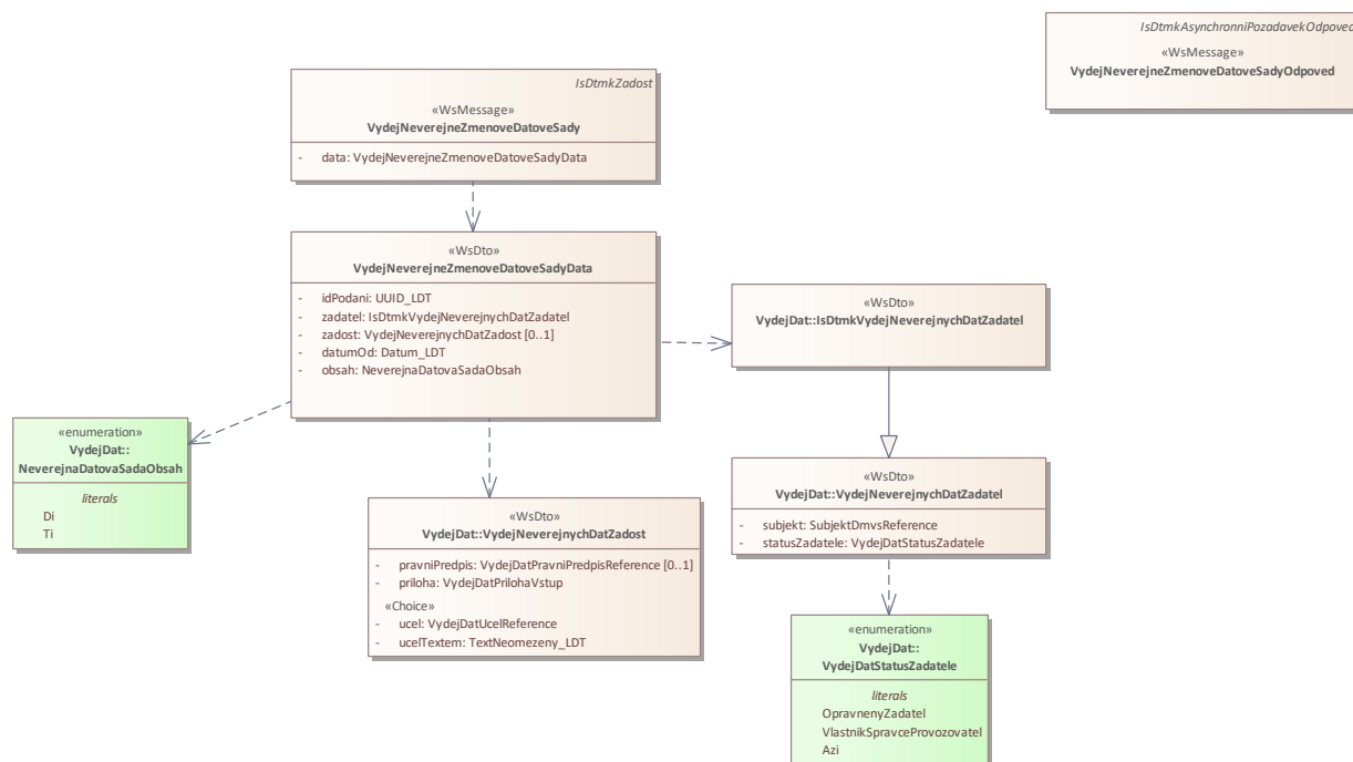
Obrázek 2. SoaML diagram pro operaci vydejNeverejneZmenoveDatoveSady
