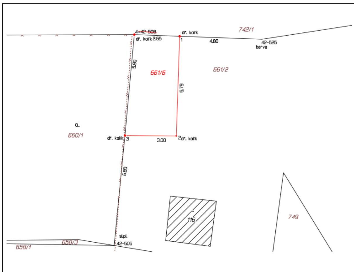
Náčrt ZPMZ č. ...., k. ú. ....
